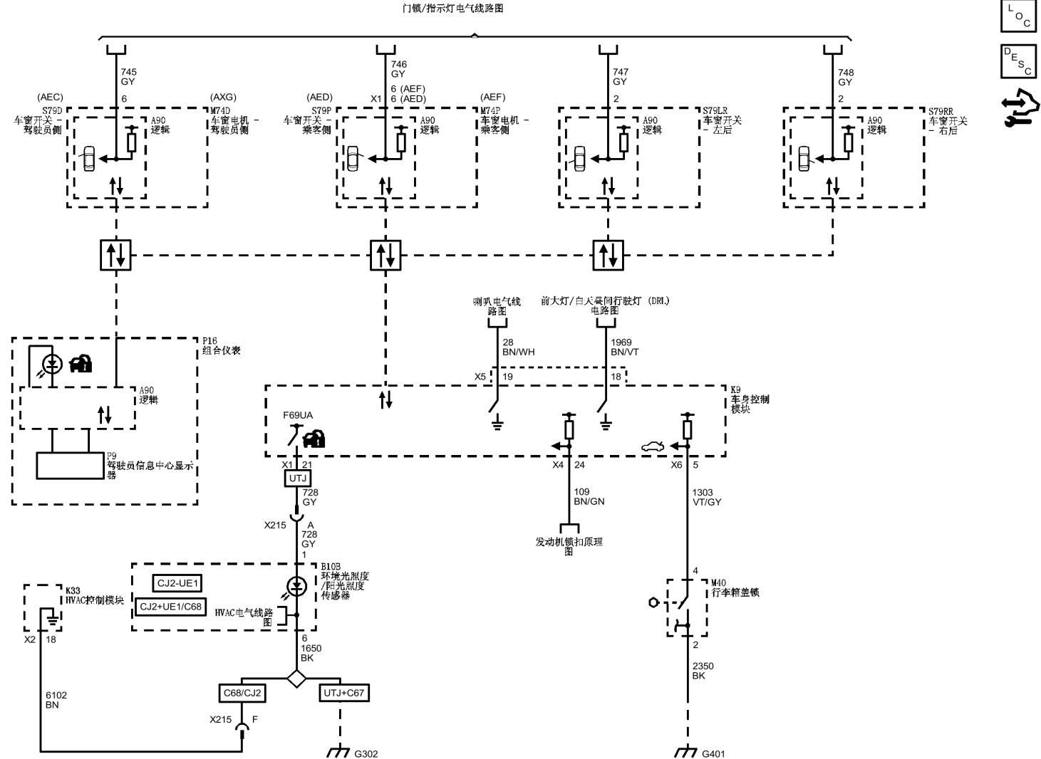
门锁/指示灯电气线路图
